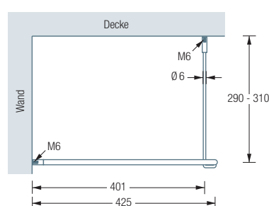
G400HD Seitenansicht:
