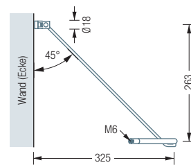
G300VW Seitenansicht:
