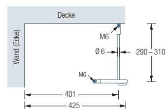
G400VD Seitenansicht:
