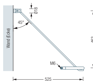
G500VW Seitenansicht:
