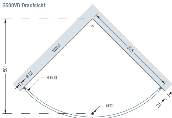
G500VD Draufsicht:
