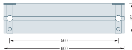
G9-600/1200 G/H/CDF/CDFF Seitenansicht:
