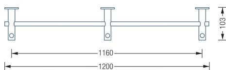
G9-1200 Draufsicht:
