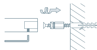
Wandmontage mit Senkhülse:
