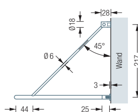
GU1-800 Seitenansicht:
