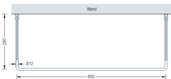
GU1-800 Draufsicht:
