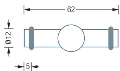
HG18-50D-B Frontansicht:
