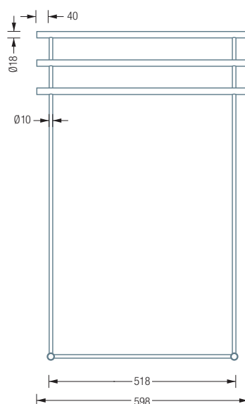
HTB3 Frontansicht:
