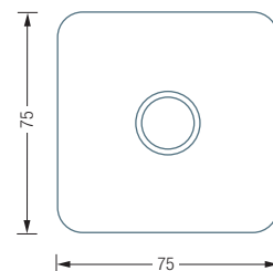
KK75S Frontansicht:
