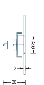
KK75S Seitenansicht:
