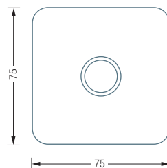
KK75S Frontansicht:
