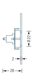
KK75S Seitenansicht:
