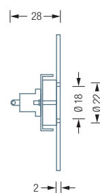
KK75R Seitenansicht:
