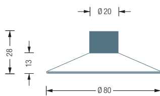
TSB80-13 Seitenansicht:
