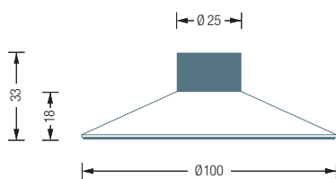
TSB100-18 Seitenansicht:
