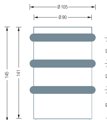
TSB90-145 Seitenansicht:
