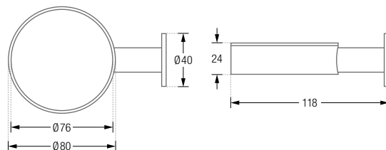
ATF Drauf- / Seitenansicht:
