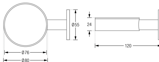
ATF-K55 Drauf- / Seitenansicht:
