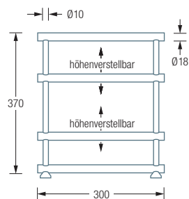
BR600-3 Seitenansicht:
