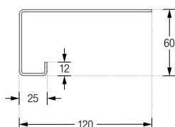
DA200H/DA300H Seitenansicht:
