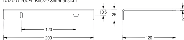
DA200 / 200PL Rück- / Seitenansicht:
