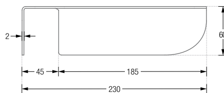
DAE230K / 230K-PL Seitenansicht:
