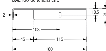
DAE160 Seitenansicht:
