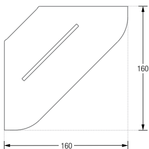
DAE160 / 160K Draufsicht:
