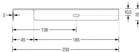
DAE230 / 230PL Seitenansicht:
