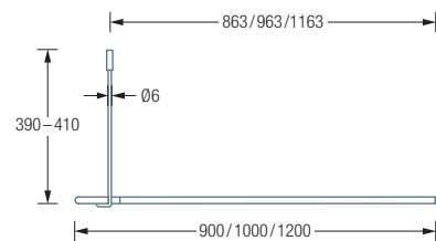
DSE900 / 1000 / 1200 Seitenansicht:
