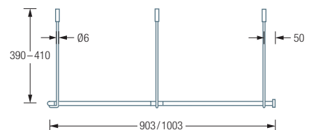
DSFE900F / 1000F Seitenansicht:
