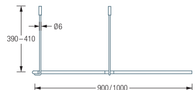
DSFE900 / 1000 Seitenansicht:
