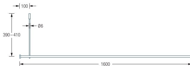
DSN12-1600DW Seitenansicht:
