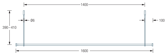
DSN12-1600F Seitenansicht:
