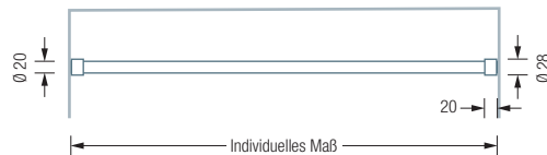
DSRN20 Frontansicht:
