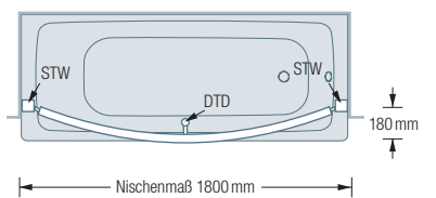
DSGN12 Draufsicht – mit Radius 1800 mm:
