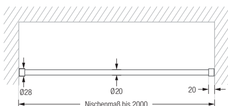
DSRN20-1/-2/-3 Frontansicht:
