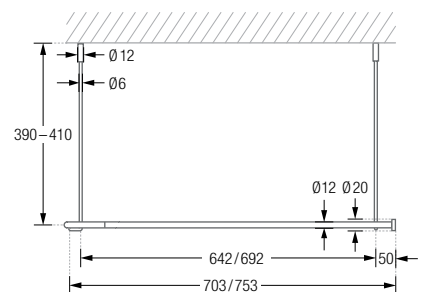
DSU1700-700F / 750F Seitenansicht:
