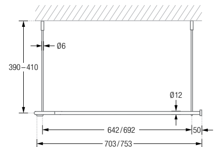
DSU1700-700F / 750F Seitenansicht:
