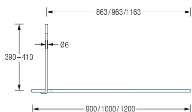
DSU900-900 / 1000-1000 / 1200-1200 Seitenansicht:
