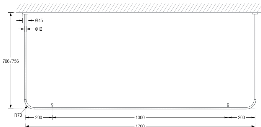
DSU1700-700K45 / 750K45 Draufsicht:
