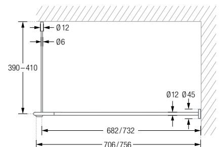
DSU1700-700K45 / 750K45 Seitenansicht:
