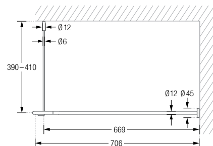
DSU1400-700K45 / 1600-700K45 Seitenansicht:
