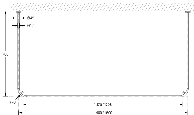
DSU1400-700K45 / 1600-700K45 Draufsicht:
