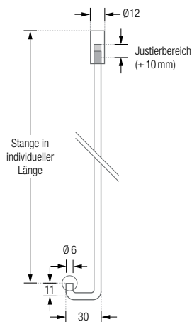
DTDM Seitenansicht:
