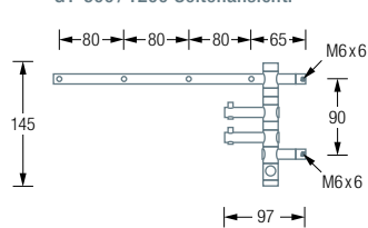
G1-600 / 1200 Seitenansicht:
