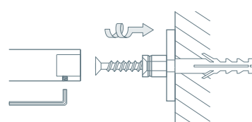
Wandmontage mit Hutrosette:
