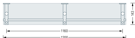
G4-1200G/H Draufsicht:
