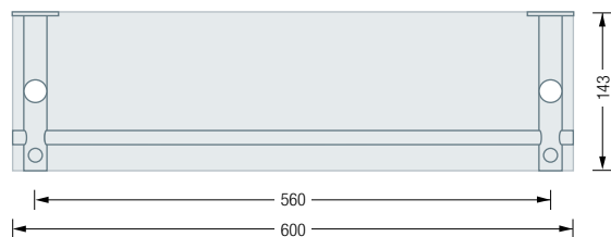
G4-600G/H Draufsicht:
