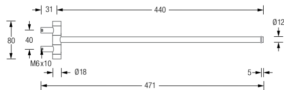
GHH2 Seitenansicht:
