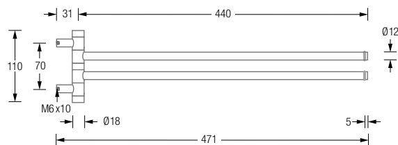
GHH2 Seitenansicht:
