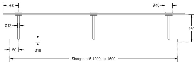
GSUN18-2 Frontansicht:
