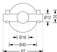
H18-50DK45-B Frontansicht:
