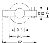
H18-50DR40-B Frontansicht:
