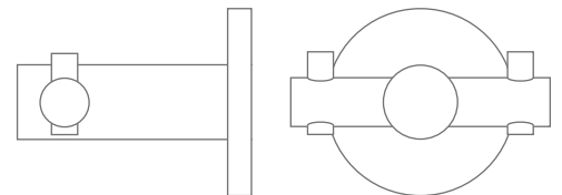
H18-50DK45 Doppel-Haken zur Verklebung Ø18 mm, Länge 56 mm, Breite 62 mm
