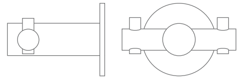
H18-50DR40 Doppel-Haken zur Verschraubung Ø18 mm, Länge 53 mm, Breite 62 mm
