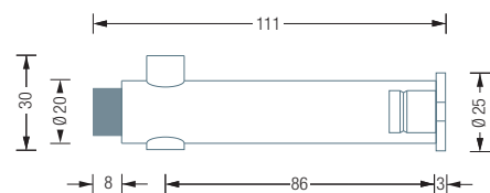
H20-100TS Seitenansicht:
