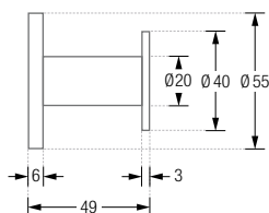
HA3-R40S55-B Seitenansicht:
