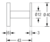
HA1-R40S40-B Seitenansicht:
