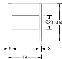
HA3-R55S55-B Seitenansicht:
