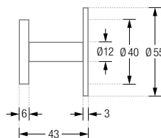
HA1-R55S40-B Seitenansicht:
