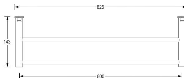
Produktbeispiel HS20-140ED800 Draufsicht:
