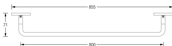
Produktbeispiel HS12-800G-K55 Draufsicht:
