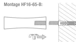
Montage HF16-65-B:
