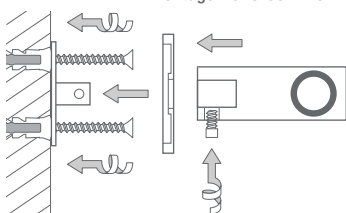
Montage HG18-50DR40-B:
