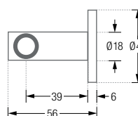
HG18-50DK45-B Seitenansicht:
