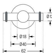
HG18-50DR40-B Frontansicht:
