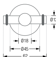
HG18-50DK45-B Frontansicht:
