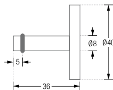
HG8-30K40-B Seitenansicht:
