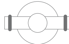
HG18-50DR40 Doppel-Haken zur Verschraubung Ø18 mm, Länge 53 mm, Breite 62 mm
