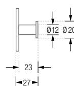
HL3H12S-B / HL5H12S-B Seitenansicht:
