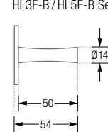
HL3F-B / HL5F-B Seitenansicht:
