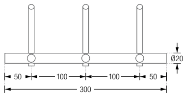
HLS3H-B Frontansicht:
