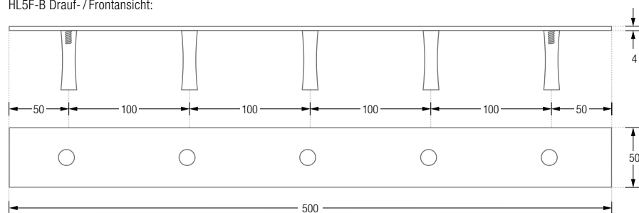
HL5F-B Drauf- / Frontansicht:
