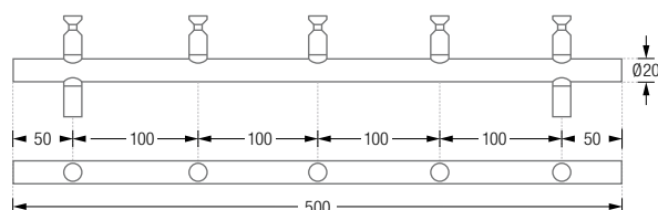
HLS5-B Drauf- / Frontansicht:
