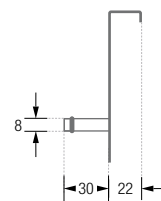
TG3-B/TG5-B Seitenansicht:
