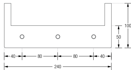
TG3-B Frontansicht:
