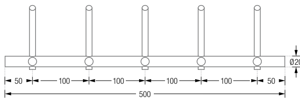
HLS5H-B Frontansicht:
