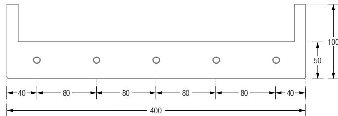
TG5-B Frontansicht:
