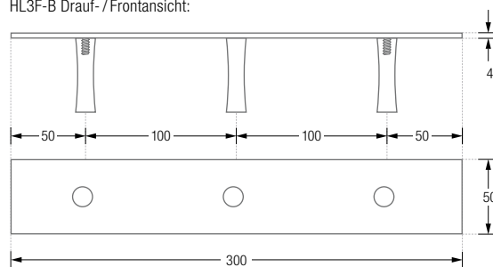
HL3F-B Drauf- / Frontansicht:
