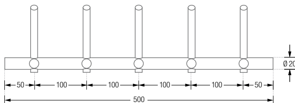
HLS5H-B Frontansicht:
