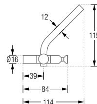
HLS3H/HLS5H Seitenansicht:
