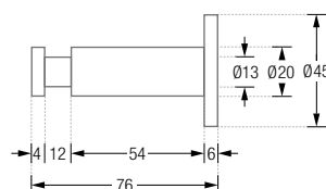
HN20-70K45 Seitenansicht:
