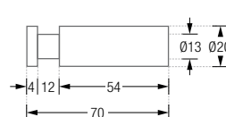
HN20-70 Seitenansicht:
