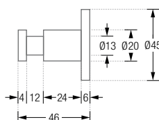
HN20-40K45 Seitenansicht:
