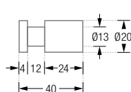
HN20-40 Seitenansicht:
