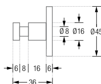
HN16-30K45 Seitenansicht:
