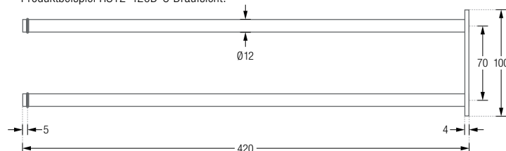
Produktbeispiel HS12-420D-0 Draufsicht:
