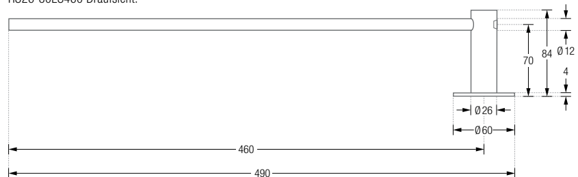
HS26-80ES460 Draufsicht:
