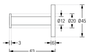
HSF1-L-K45-B:
