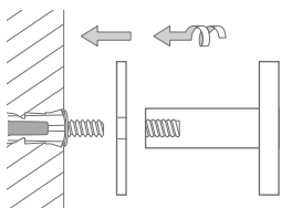
Montage HSF3-K-R40-B:
