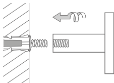
Montage HSF3-K-R40-B:
