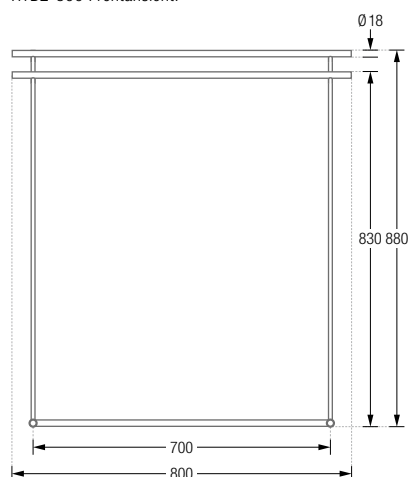
HTB2-800 Frontansicht:
