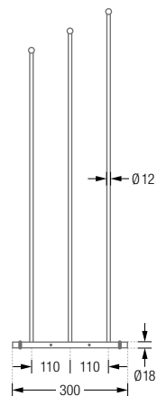
HTB3-600/800 Seitenansicht:
